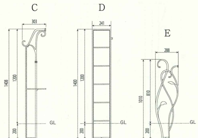
■施工寸法図 (単位:mm)
